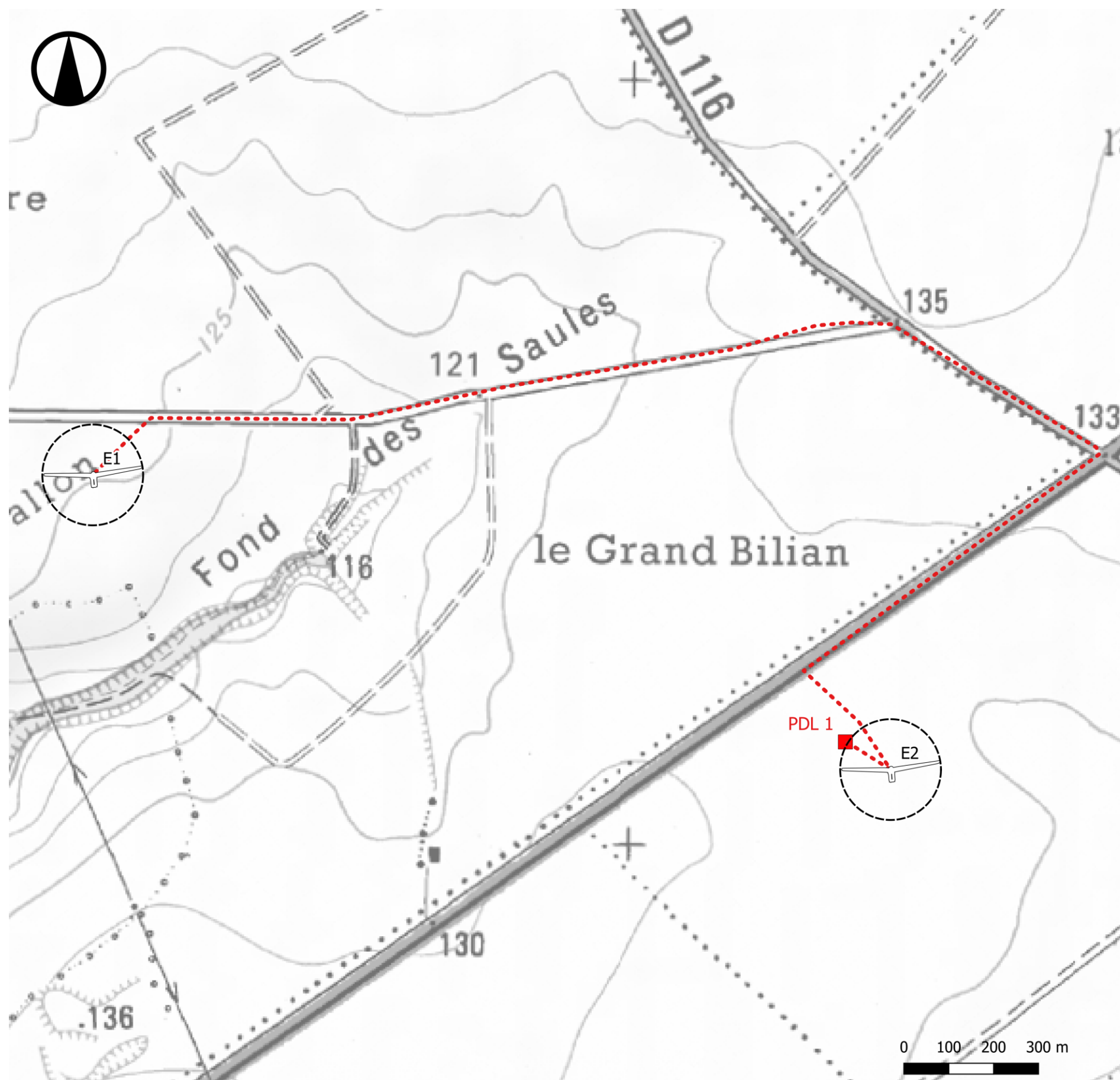
Carte 12 : Raccordement inter-éolien
